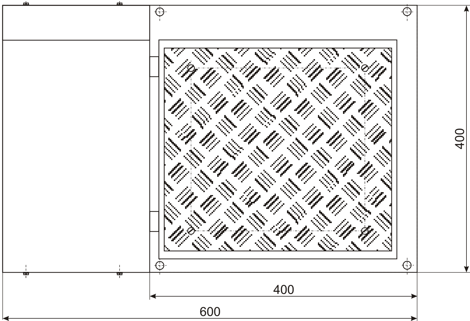
Szarpak typ US-351 (gabaryty)
